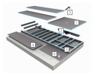
C Systemaufbau Sockelkonstruktion
