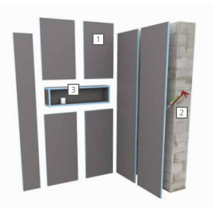
A Systemaufbau Duschwandlösung
